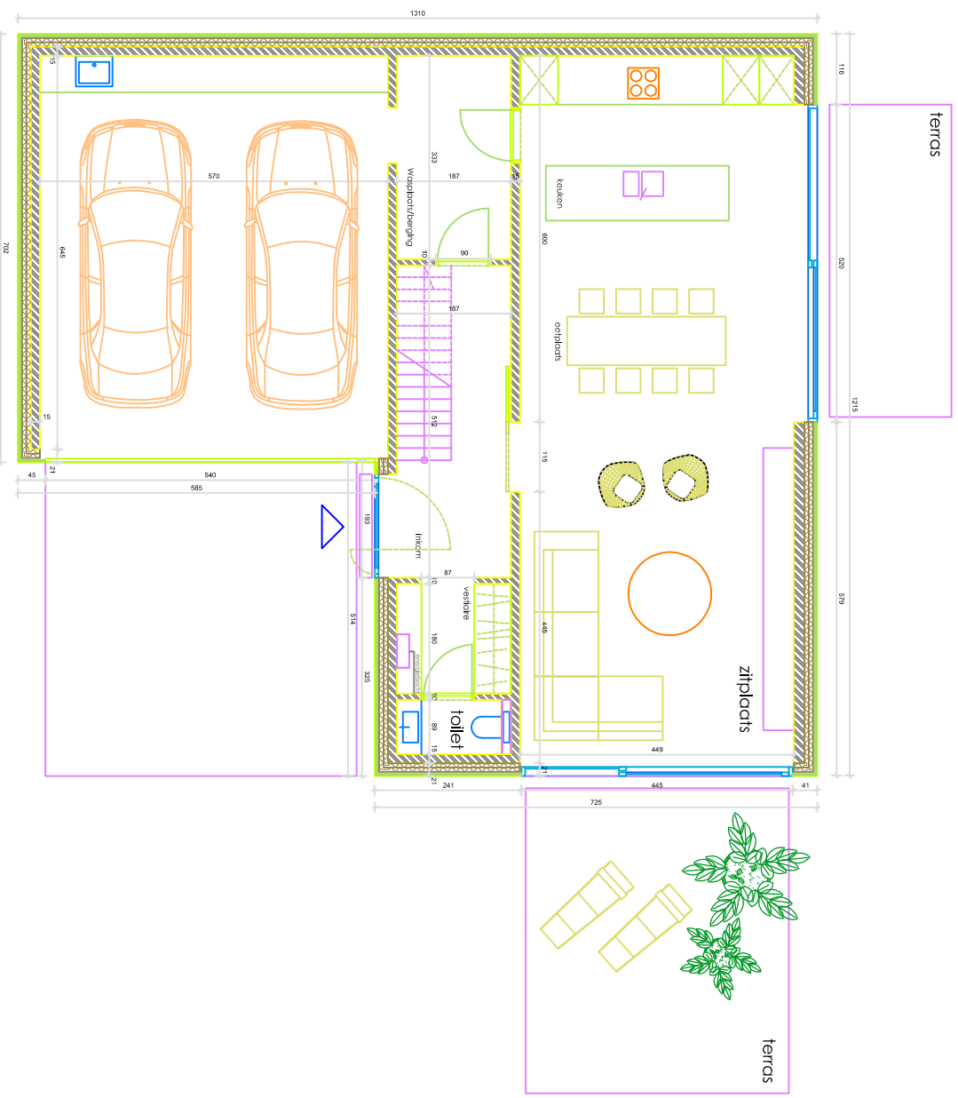
plan GELIJKVLOERS - Vrijstaande Woning * Woonref Ljda VII *
