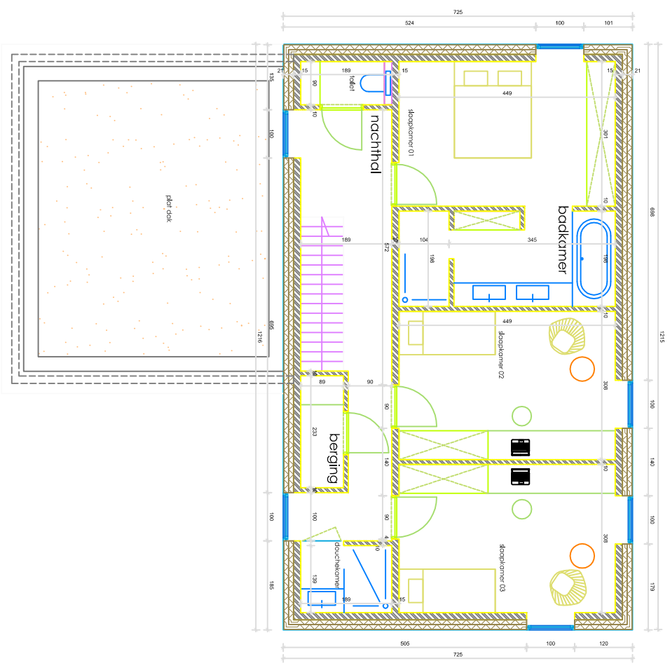
plan VERDIEPING - Vrijstaande Woning * Woonref Ljda VII *
